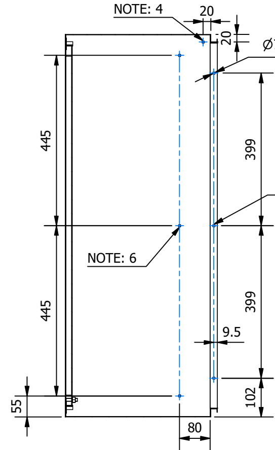
SECTION D-D
