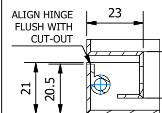
DOOR HINGE SECTION
